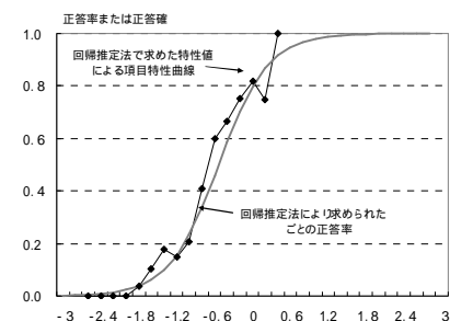
【図 4】回帰推定法によって推定した項目特性値による項目特性曲線と実際の正答率
