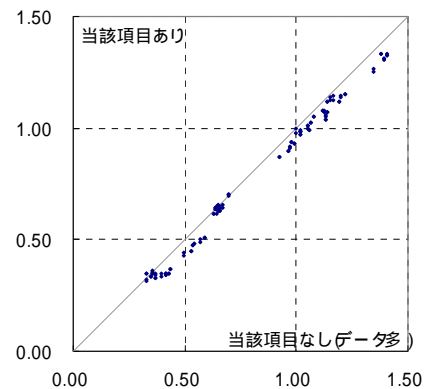
【図8】回帰分析法で特性値を推定する際に，当該項目を抜いて算出した \beta をもとにした場合と当該項目を含めたまま算出した \beta をもとにした場合の比較
