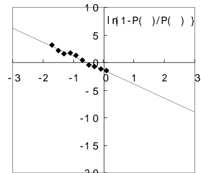
【図 3】回帰推定法による項目特性値の推定 直線の傾きと切片から項目特性値が推定できる
