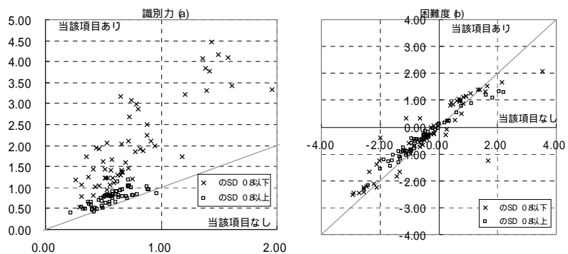
【図8】回帰分析法で特性値を推定する際に，当該項目を抜いて算出した \beta をもとにした場合と当該項目を含めたまま算出した \beta をもとにした場合の比較
