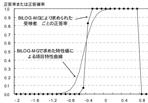
【図 2】BILOG-MG で求めた項目特性値( a=5.52 , b=-0.49 )による項目特性曲線と のレベルごとの実際の正答率
